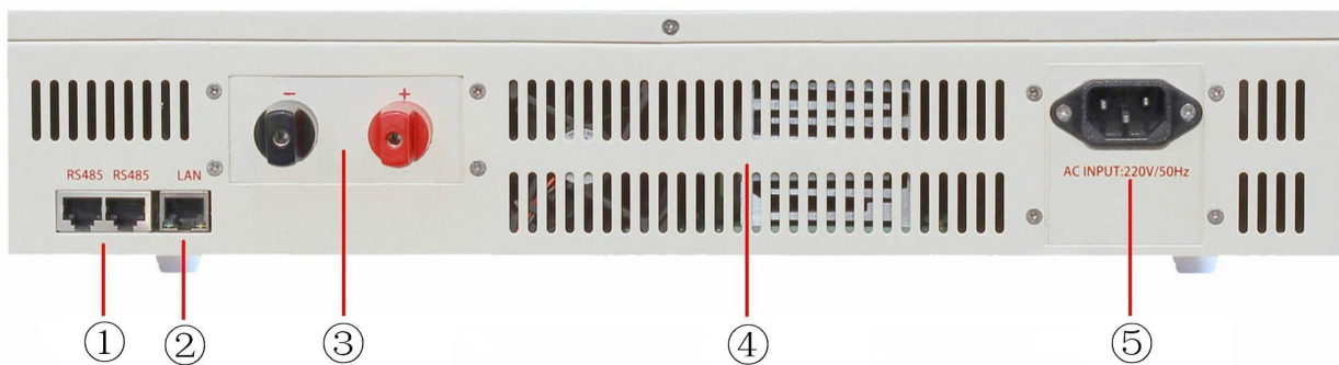
①RS-485/RS-422 通信接口 ②LAN 通信接口 ③输出接口 ④散热窗 ⑤市电输入口
