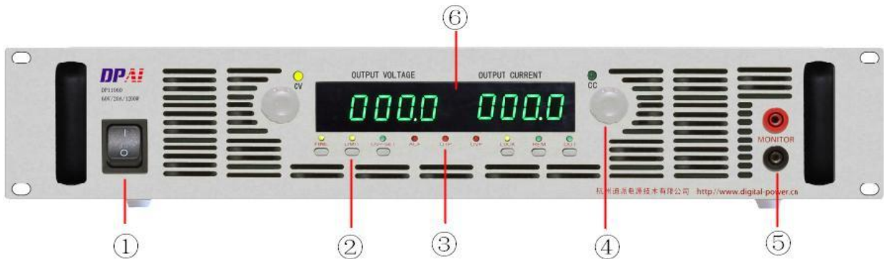
①电源开关 ②功能按键 ③状态指示 ④调节区域 ⑤输出检测 ⑥数码显示区域
