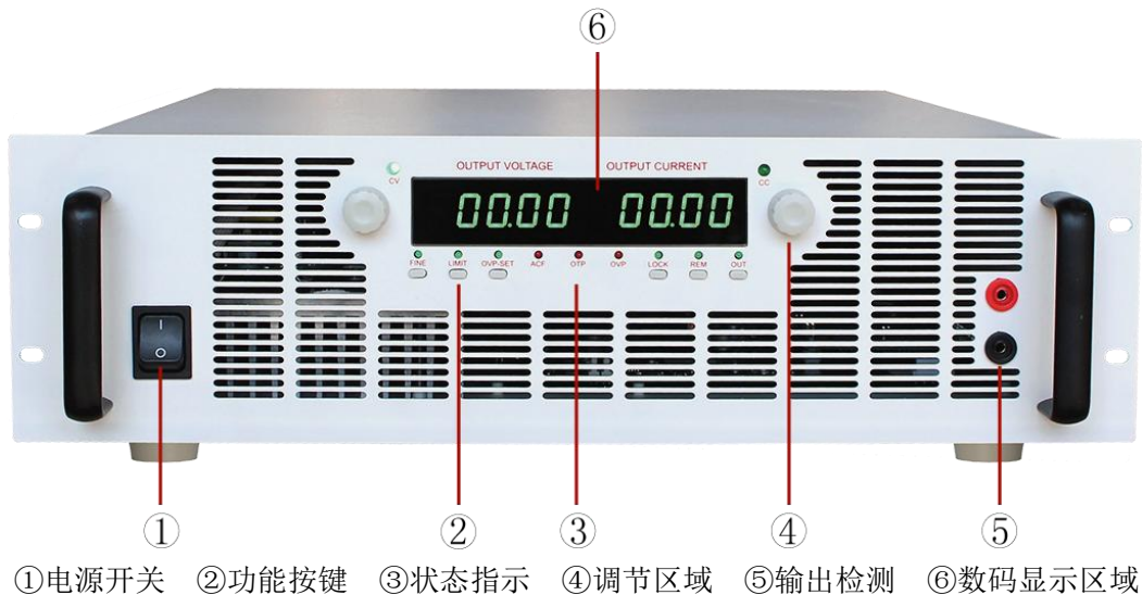
图 1 电源前面板
