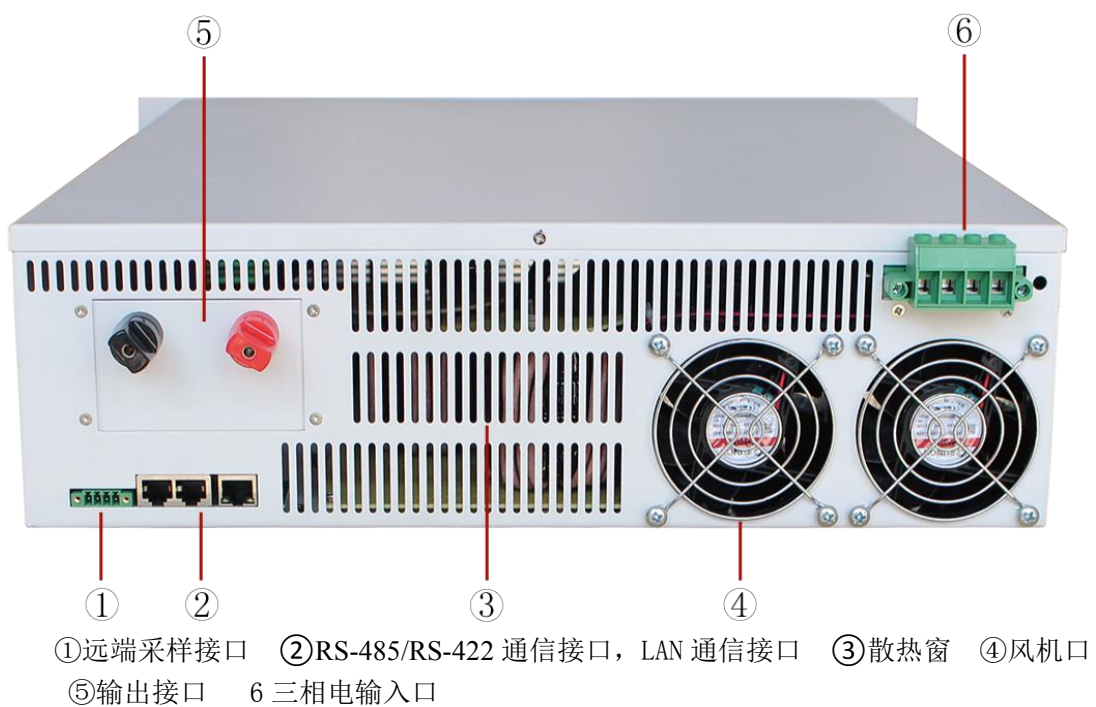
图2 电源后面板
